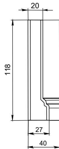
Уголок внутренний для цоколя
