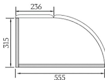
Радиусный модуль нижней базы
