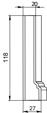
Переходник цоколя прямой
