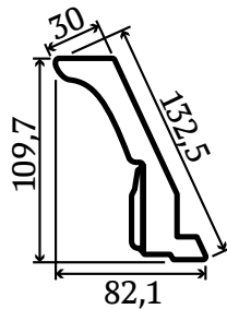
Карниз Аль Риальто полукруглый
