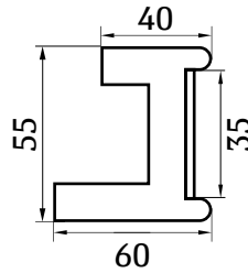
Карниз нижний полукруглый
