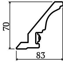
Карниз верхний полукруглый
