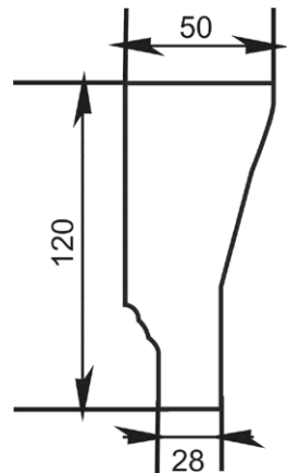
Ножка цоколя пилястры
