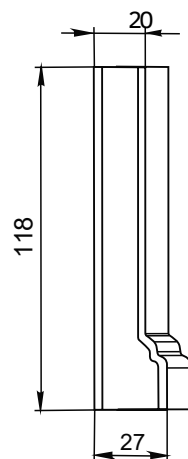
Переходник цоколя прямой
